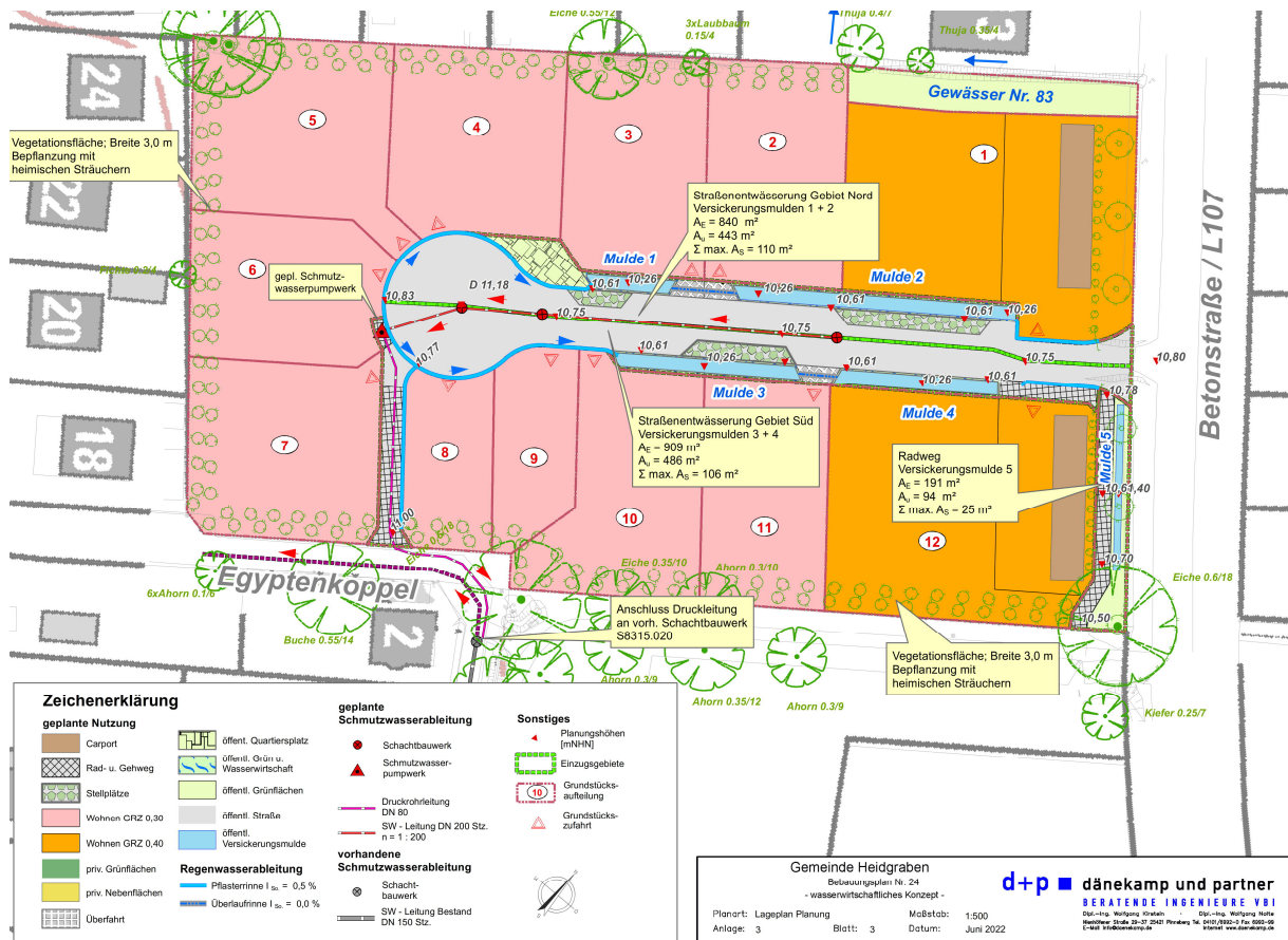
Abbildung 12 - Lageplan Entwässerung Dänekamp und partner, Anlage 3, Blatt 3
