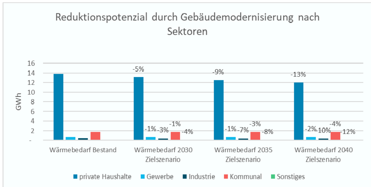
Abbildung 20 Reduktionspotenzial durch Gebäudemodernisierung nach Sektoren
