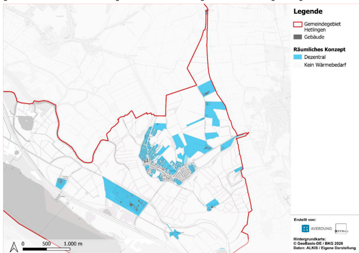
Abbildung 33: Dezentrale Gebiete
